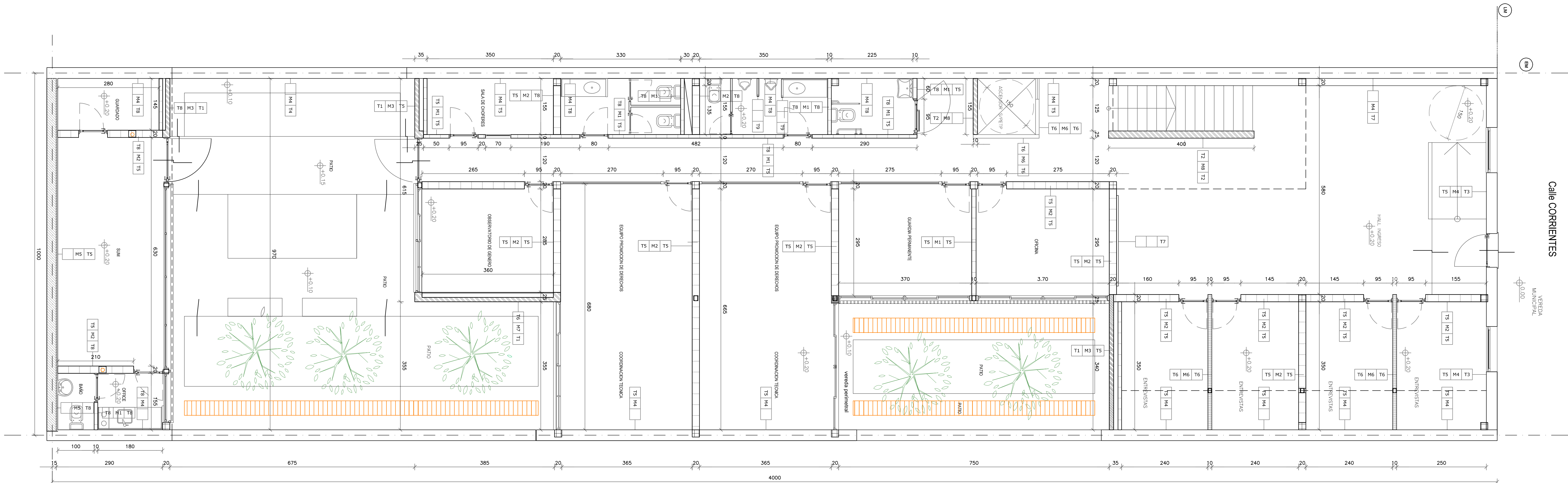
PLANTA BAJA
